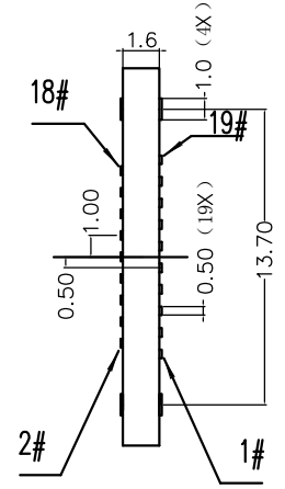
P.C.B LAYOUT
