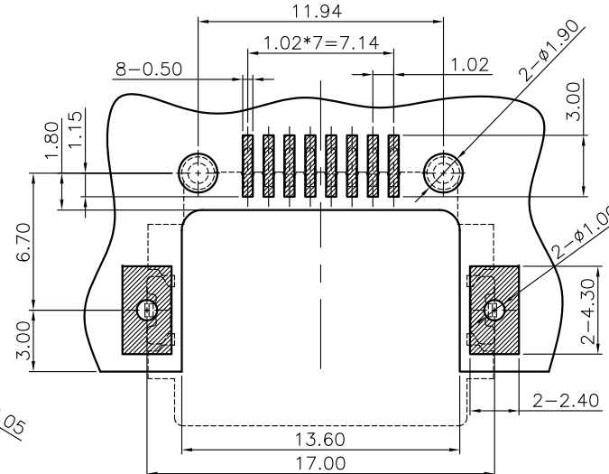
PCB LAYOUT(TOLERANCE±0.05)
